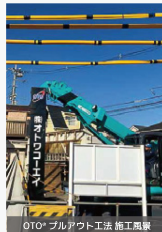
OTO® ミニロック工法 施工風景
